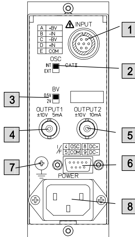
図2 - 2 : 5683 / 5684本体背面
