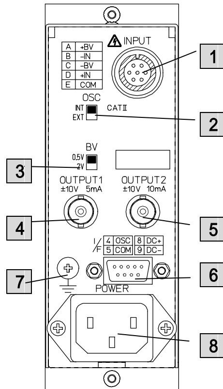
図2-7 : 5683 / 5684本体背面
