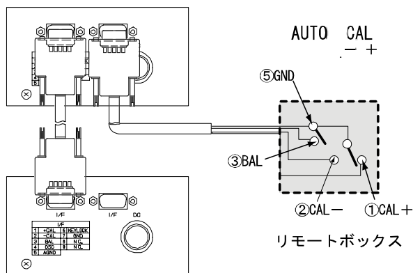
図3 - 10 リモートボックスの概略図
