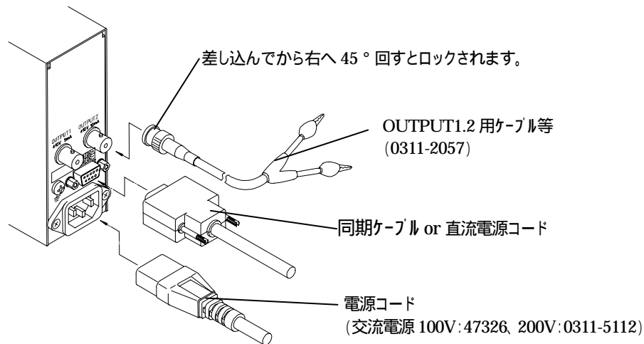
図3-2 電源、出力ケーブルの接続
