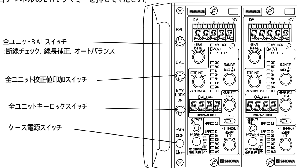
図3 - 9 ケース正面図
