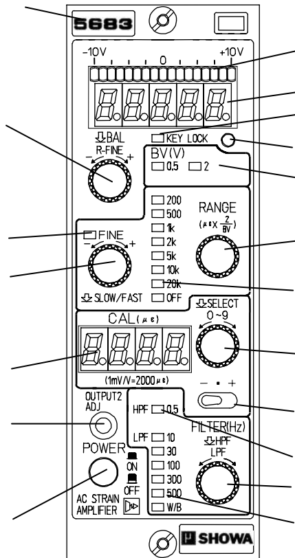
図2 - 1 : 5683 / 5684本体前面
