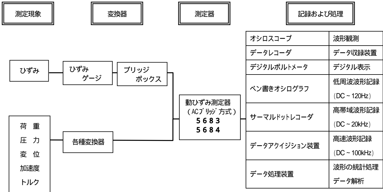
図1-1 計測ブロック図
