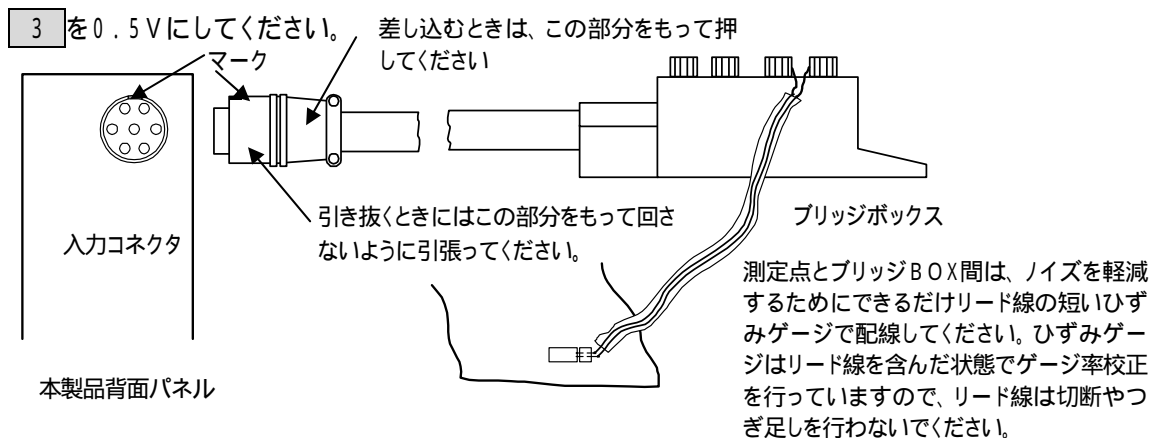
図3-1 ブリッジボックスとの接続
