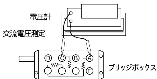
図4 - 8 ブリッジ部の電圧測定
