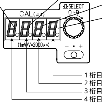
図2 - 3 校正値 (CAL) の設定
