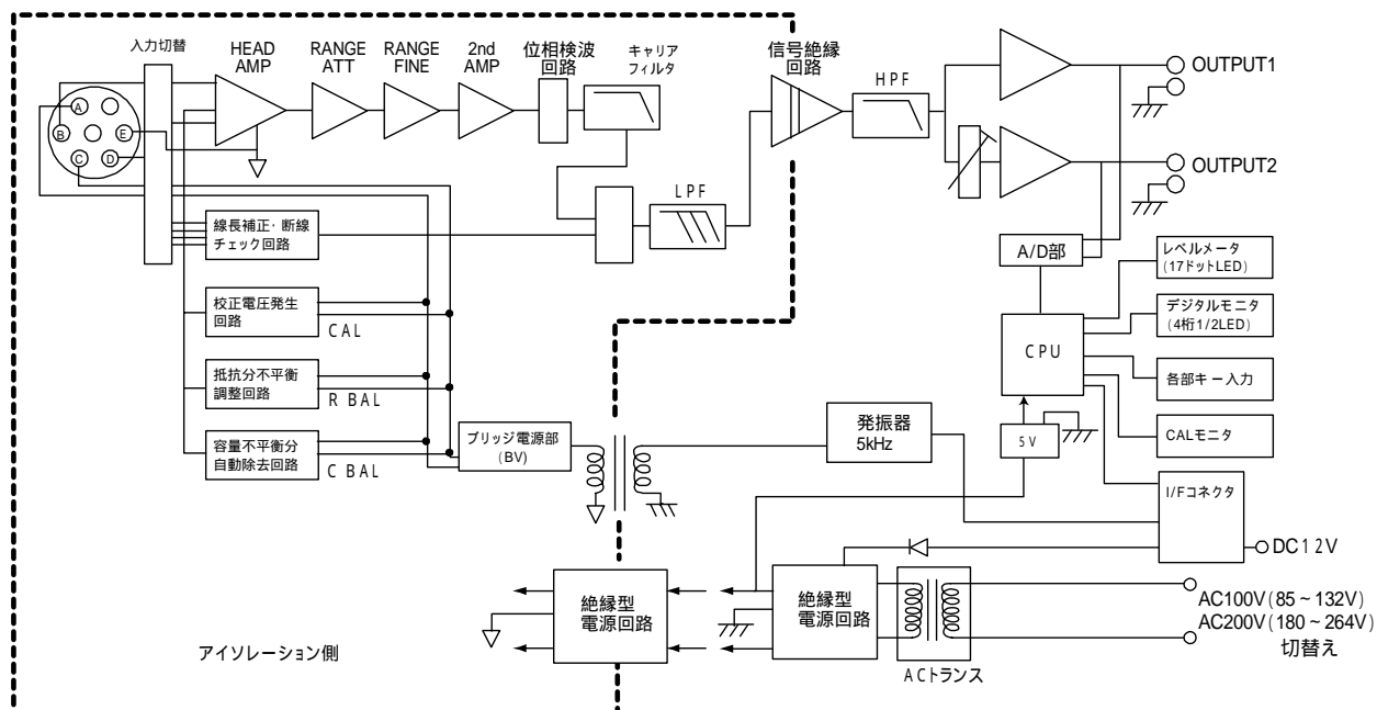
図5 - 1 ブロック図
