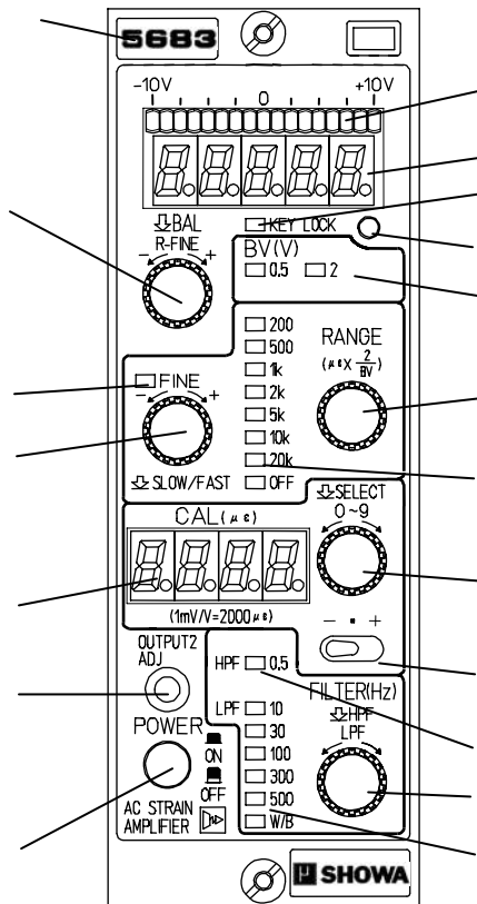
図2-6 : 5683 / 5684本体前面
