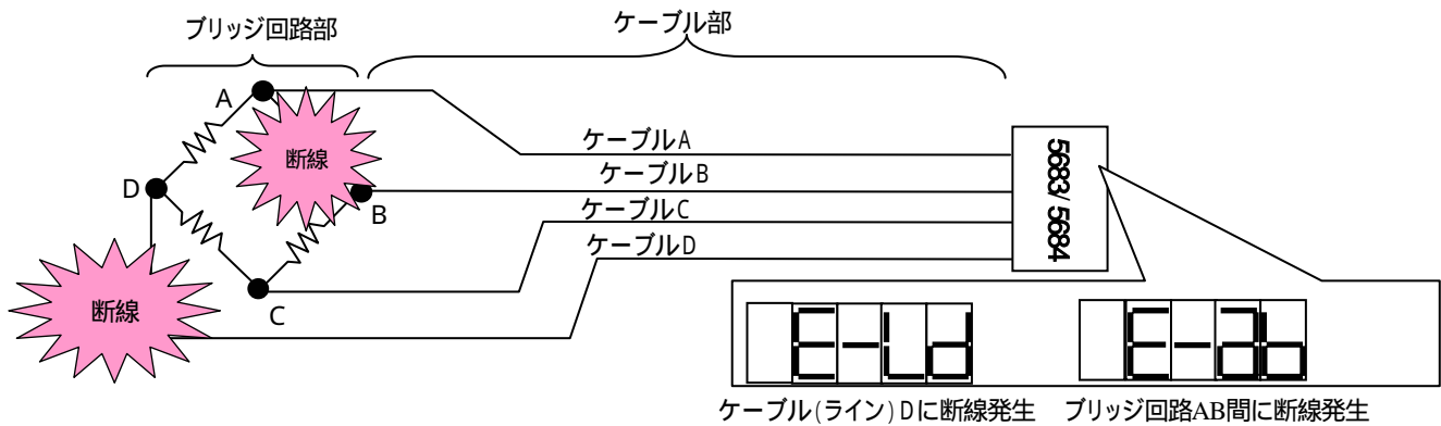
図3-3 断線チェック概略図
