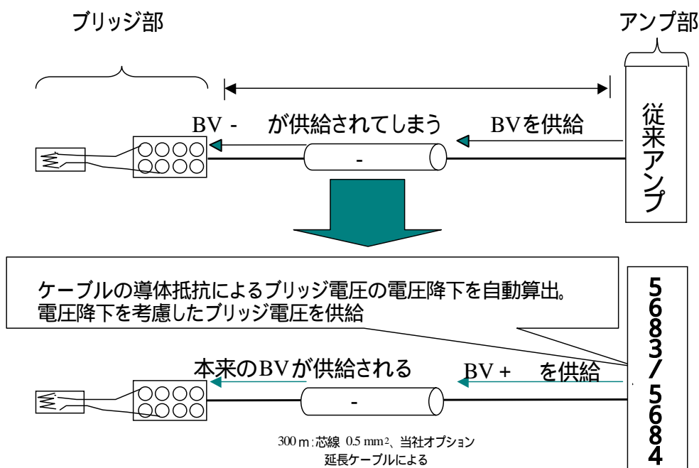
図3 - 4 線長補正機能の概略図
