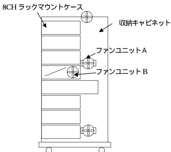
図3 - 13 ファンの配置箇所
