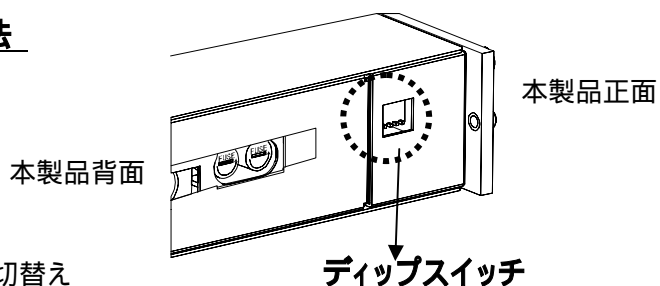
図3 - 5 ディップスイッチの位置
